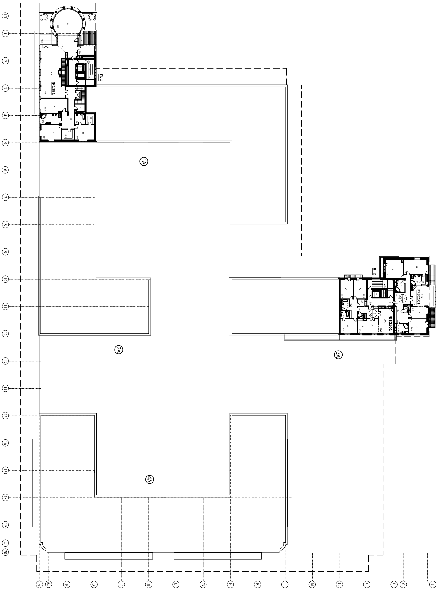
Жилой комплекс. Сводный план 10 этажа. М 1:200
